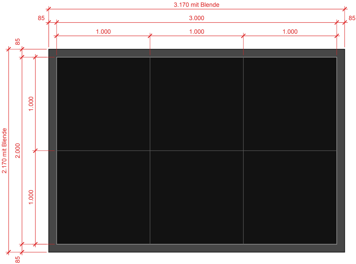
Vorderansicht außen 1:25 6 Kabinette 1.000 × 1.000 mm, 3 breit × 2 hoch
