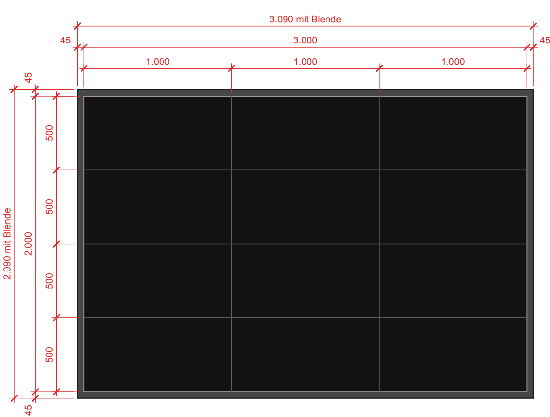
Vorderansicht innen 1:25 12 Kabinette 1.000 × 500 mm, 3 breit × 4 hoch
