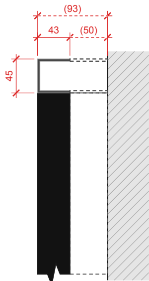
Detail A · innen Schnitt Oberkante 1:5, Ansichtsseite links
