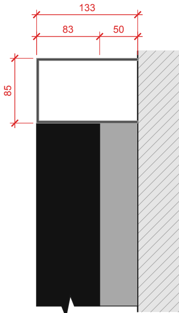
Detail B · außen Schnitt Oberkante 1:5, Ansichtsseite links
